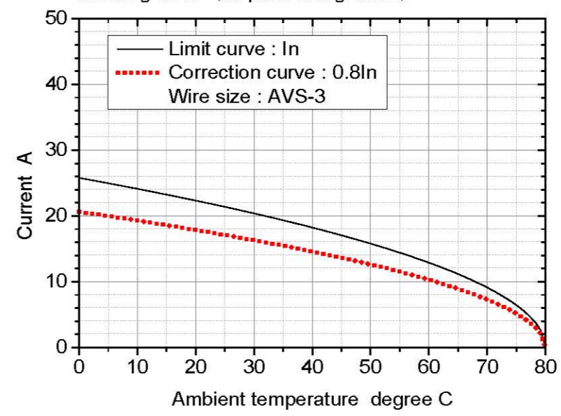
軽減曲線 (全極通電)
