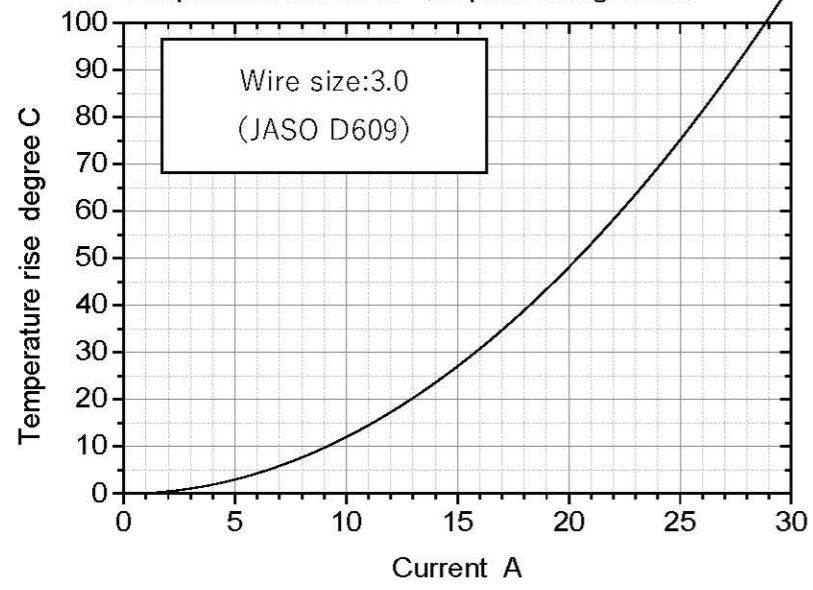
温度上昇曲線 (全極通電)
