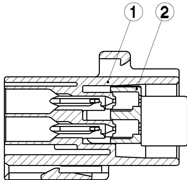
SEC. A-A
