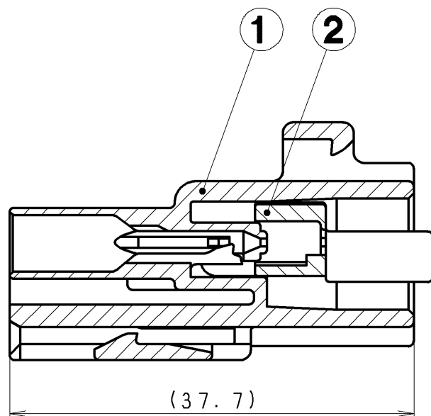
SEC. A-A
