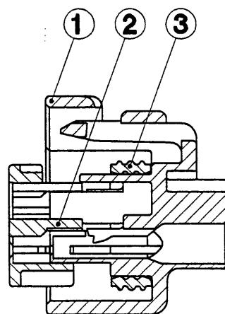
SEC. A-A
