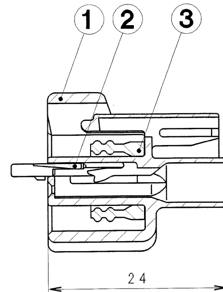
SEC. A-A
