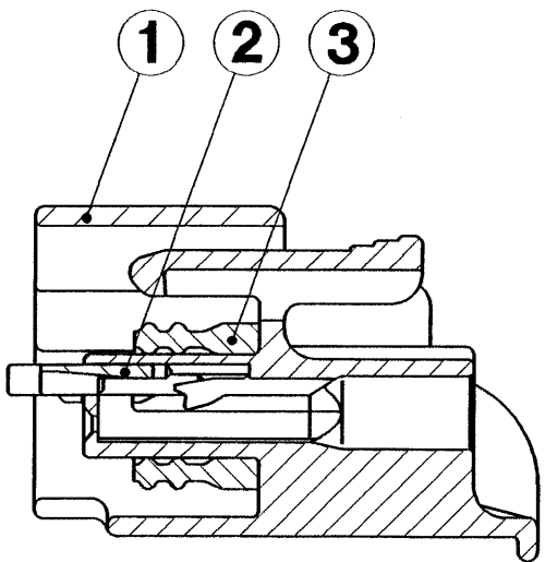
SEC. A-A
