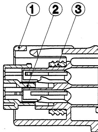
SEC. A-A
