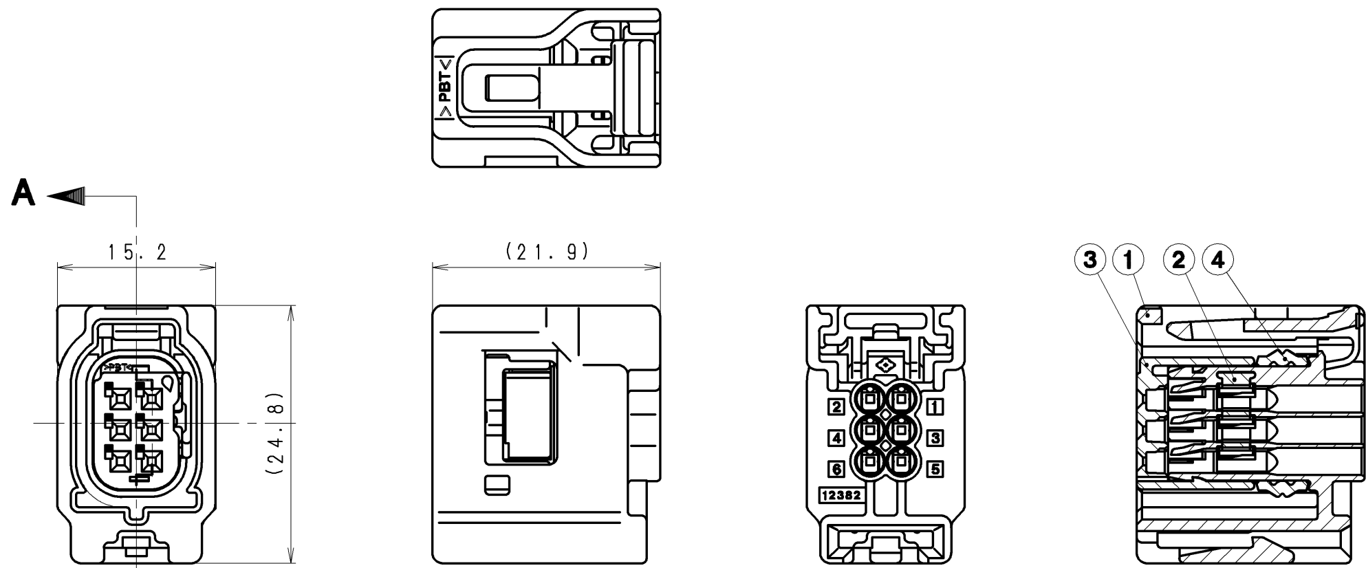
SEC. A- A
