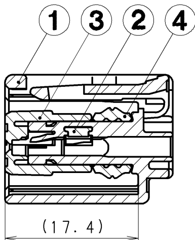
SEC. A-A
