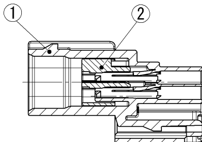
SEC. A-A
