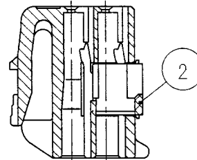
SEC. A-A
