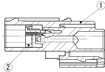
SEC. A-A
