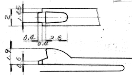
"C"部 DETAIL 5/1
