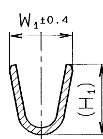
SEC. A-A
