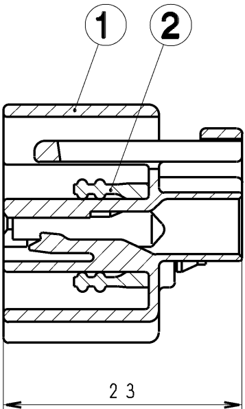
SEC. A-A
