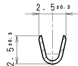
SEC A-A
